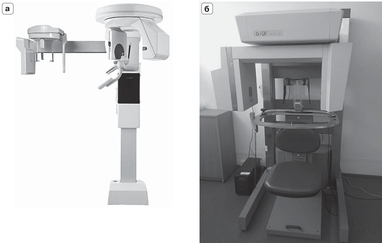
Рис. 1. Рентгенодиагностическое оборудование. а – цифровой ортопантомограф STRATO 2000; б – конусно-лучевой компьютерный томограф i-Cat.
